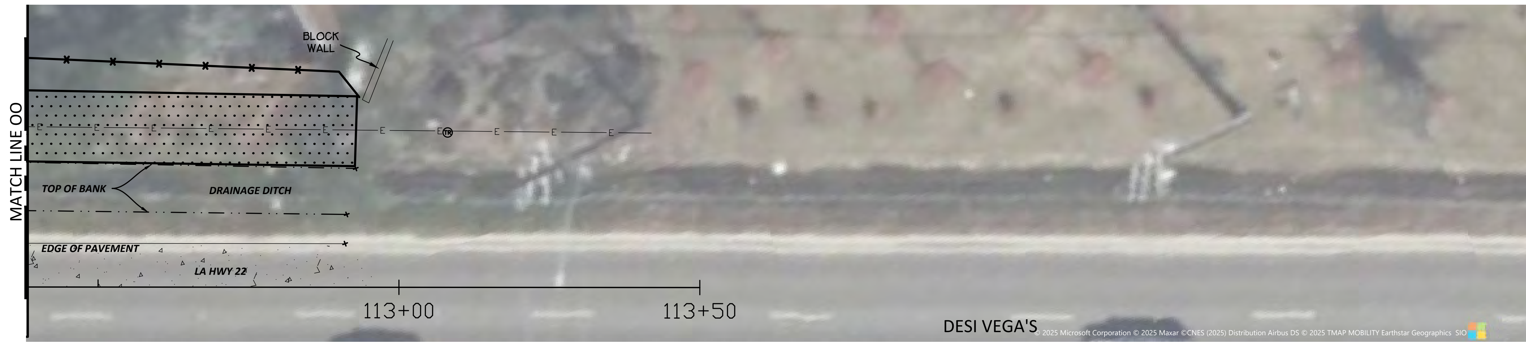
D15.0 - DEMOLITION PLAN (BASE BID)
