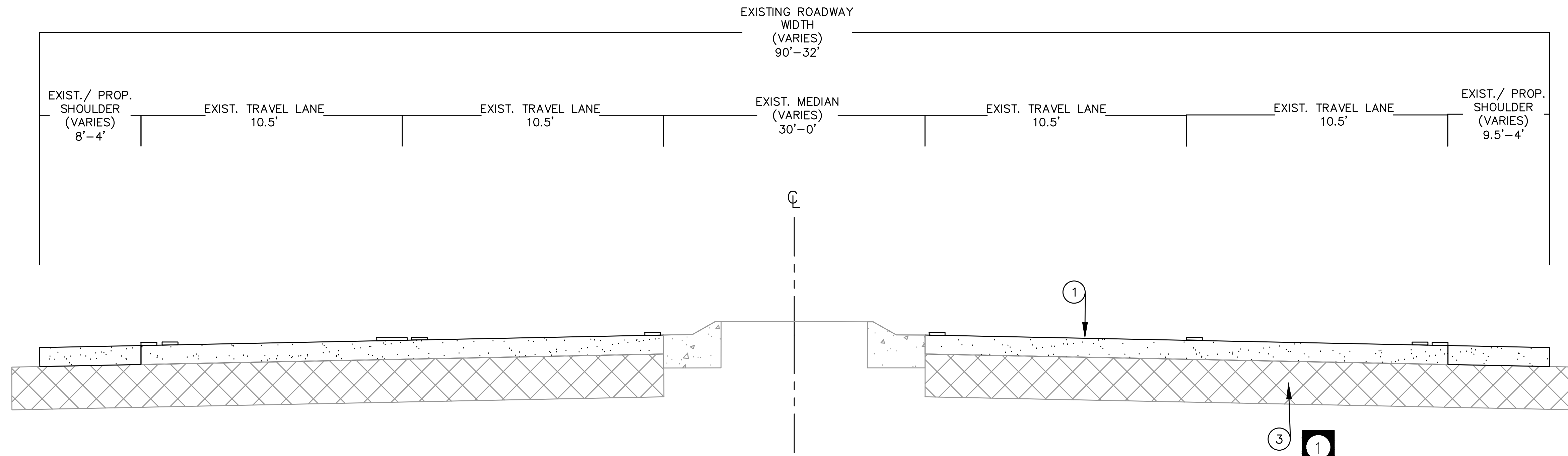
TYPICAL SECTION (N.T.S.) APPLIES TO STA 10+39 TO 21+63
