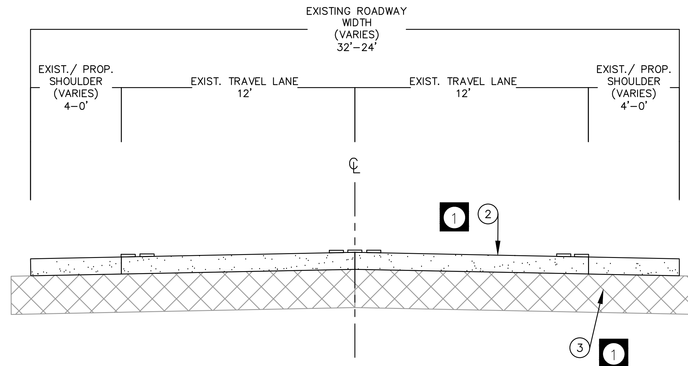
TYPICAL SECTION (N.T.S.) APPLIES TO STA 21+63 TO 187+17
