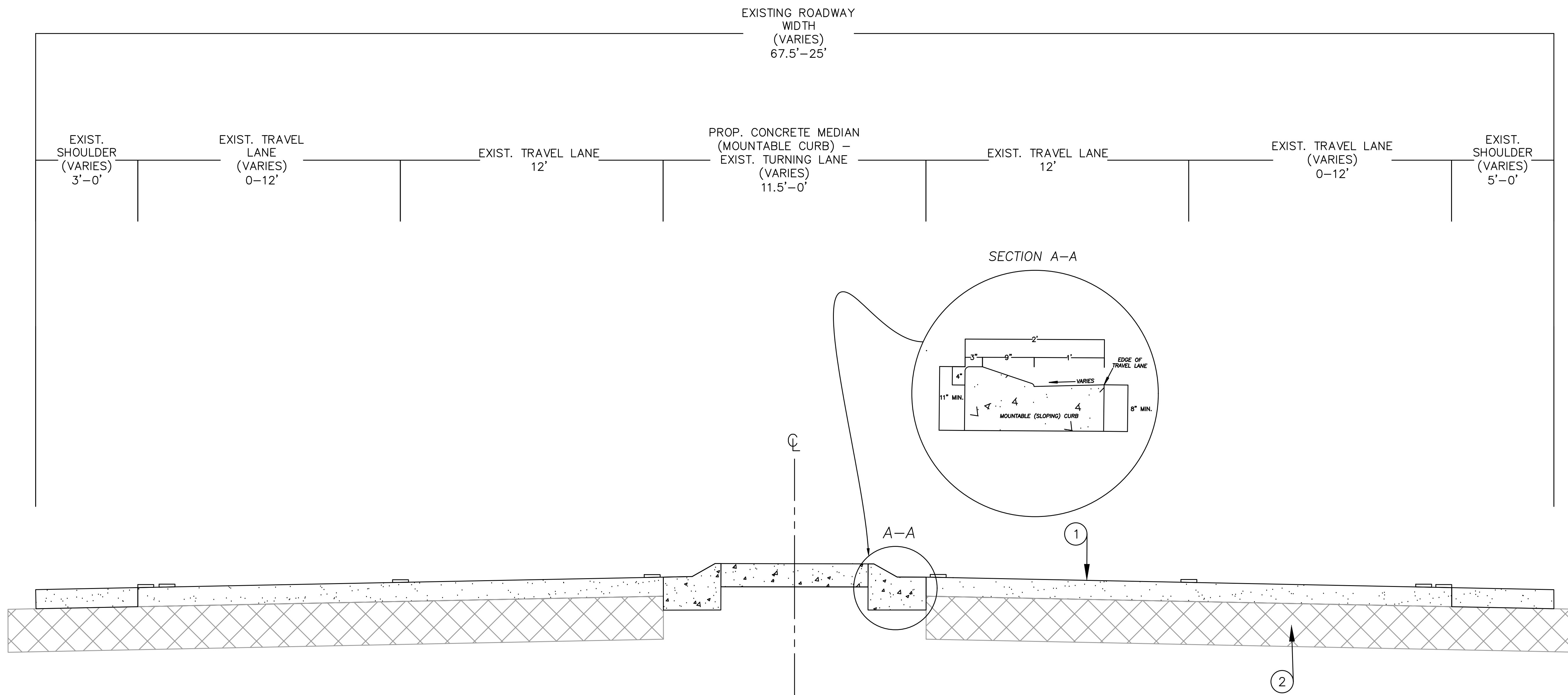
TYPICAL SECTION (N.T.S.) APPLIES TO STA 187+17 TO 240+84
