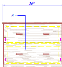
FRONT ELEVATION SCALE: 1" = 1'-0"
