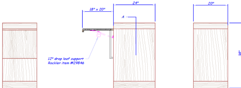
FRONT ELEVATION SCALE: 1" = 1'-0"
