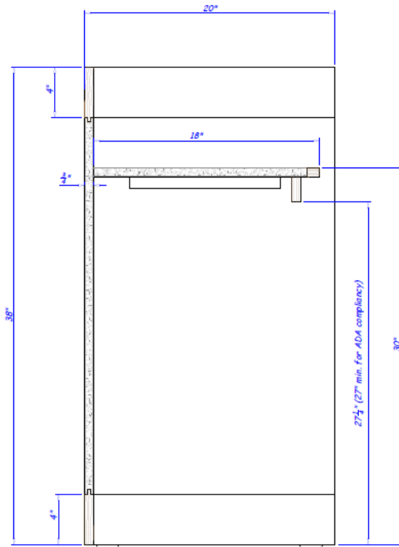
VERTICAL SECTION "A" SCALE: 3" = 1'-0"
