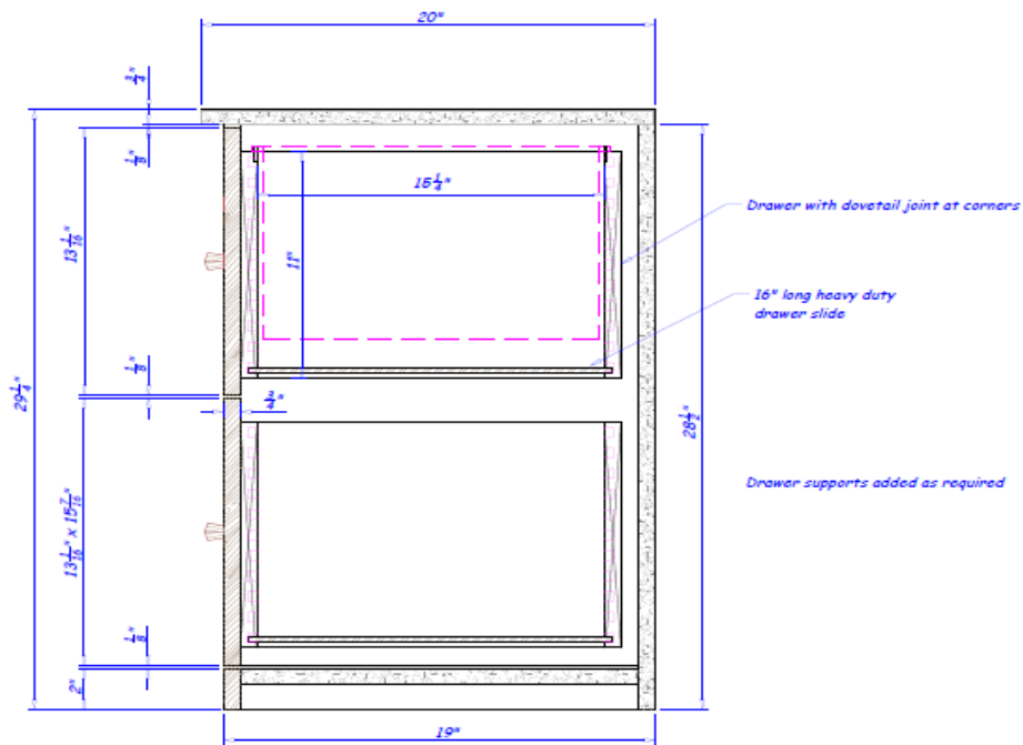
VERTICAL SECTION "A" SCALE: 3" = 1'-0"
