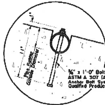
INSET "A"
