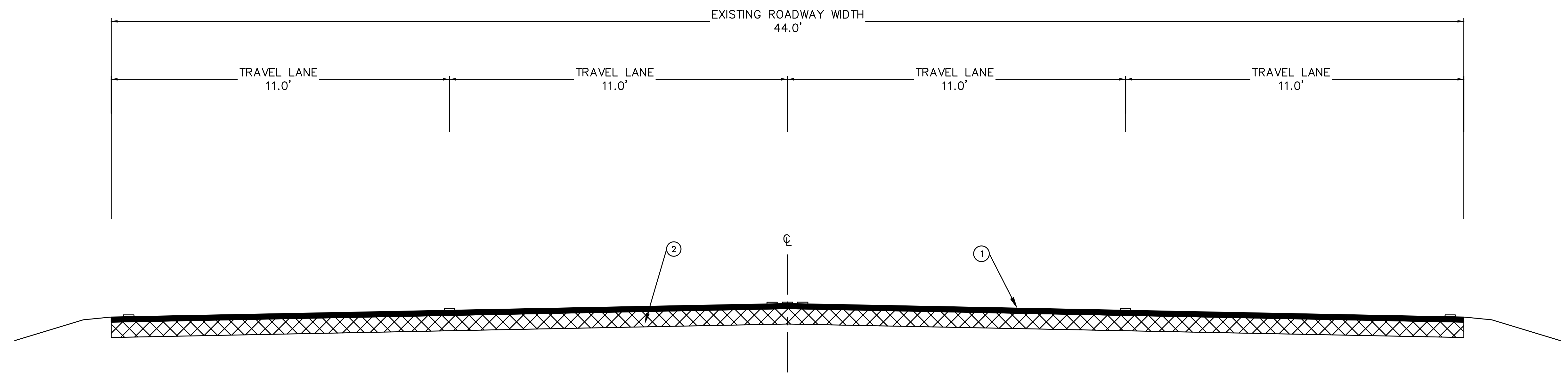
TYPICAL SECTION (N.T.S.) APPLIES TO STA 11+80 TO 15+00
