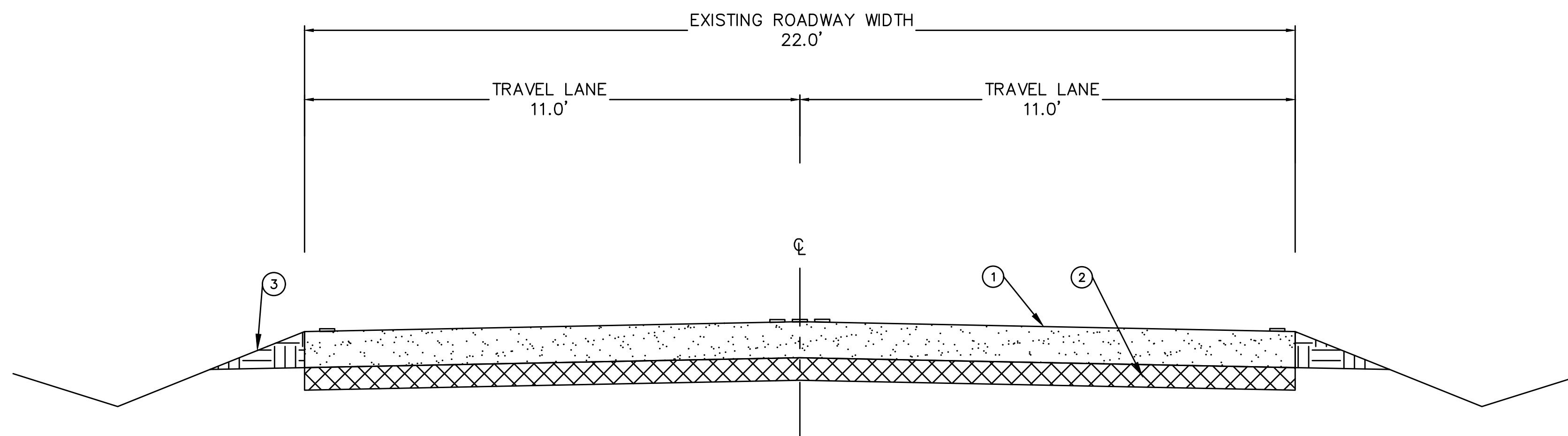
TYPICAL SECTION (N.T.S.)
