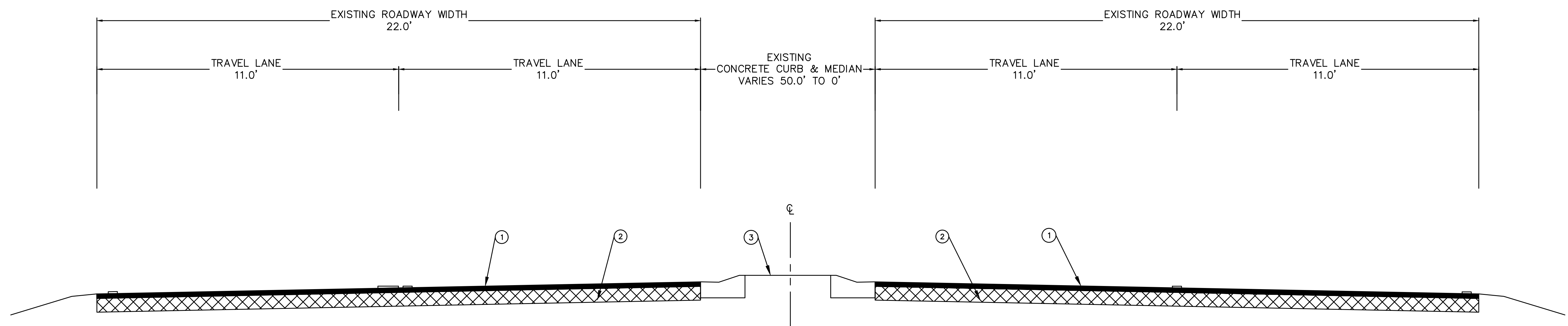
TYPICAL SECTION (N.T.S.) APPLIES TO STA 10+30 TO 11+80
